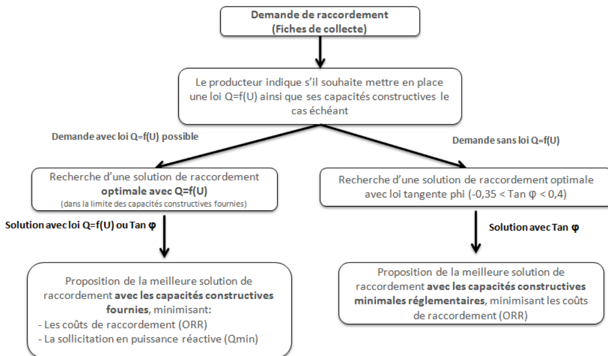
Principe de l'étude de raccordement
